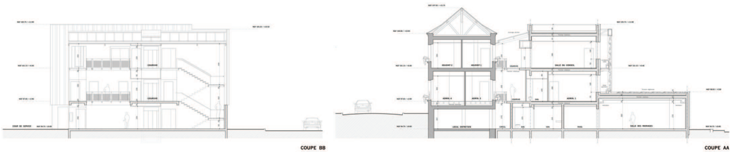
COUPE BB
