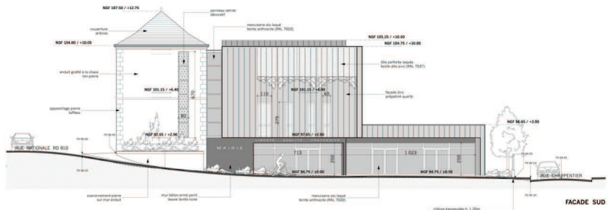
FAÇADE SUD
